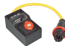
Š x V x H: 160 x 280 x 133 mm Istiacie prvky sú inštalované pod priehľadným krytom odolným voči nárazom; v tejto polohe je odolný voči striekajúcej vode
