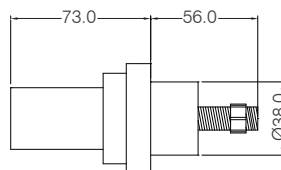
Rozmery zabudovateľnej zástrčky v mm
