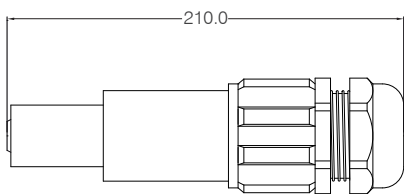
Rozmery zástrčky v mm
