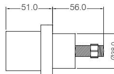
Rozmery zabudovateľnej zástrčky v mm
