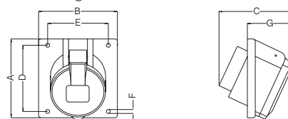
Celogumové zabudovateľné CEE zásuvky
