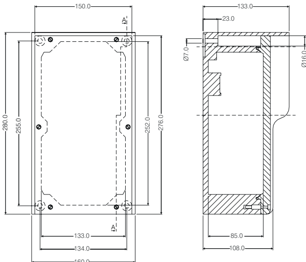
Konštrukčný rad 7250
