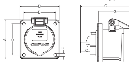
Plastové zabudovateľné CEE zásuvky, priame
