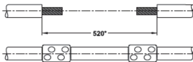
Opravná spojka
