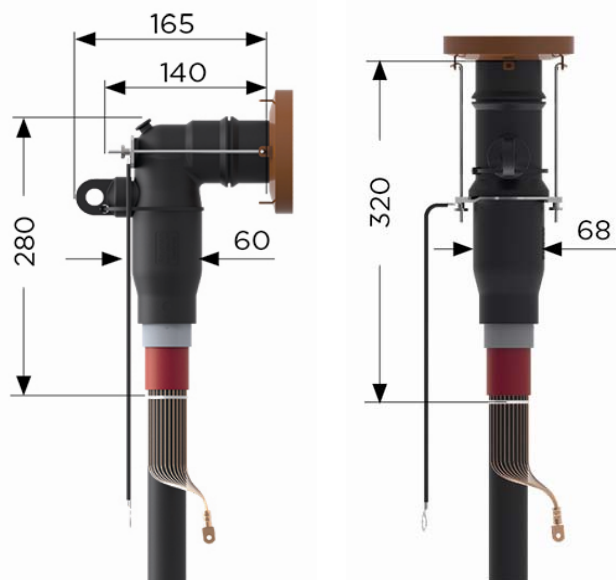
RSES-VD: Uhlový konektor s kapacitným meracím bodom
